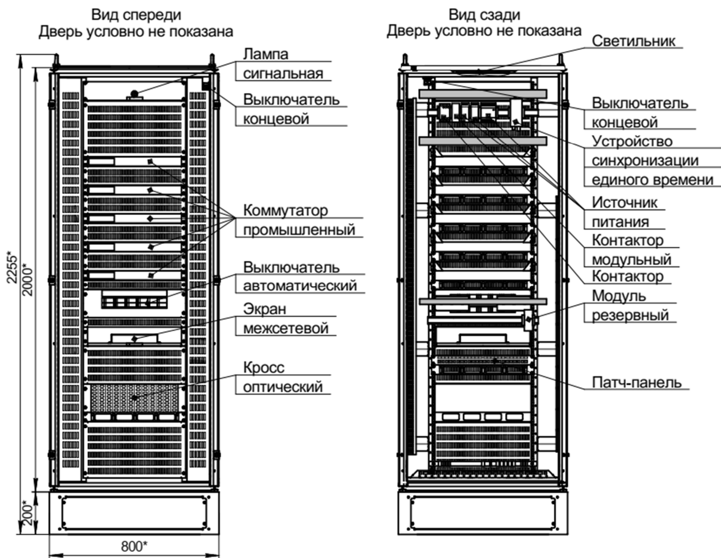
Рисунок 1. Общий вид и размеры шкафа № ЗНИ
